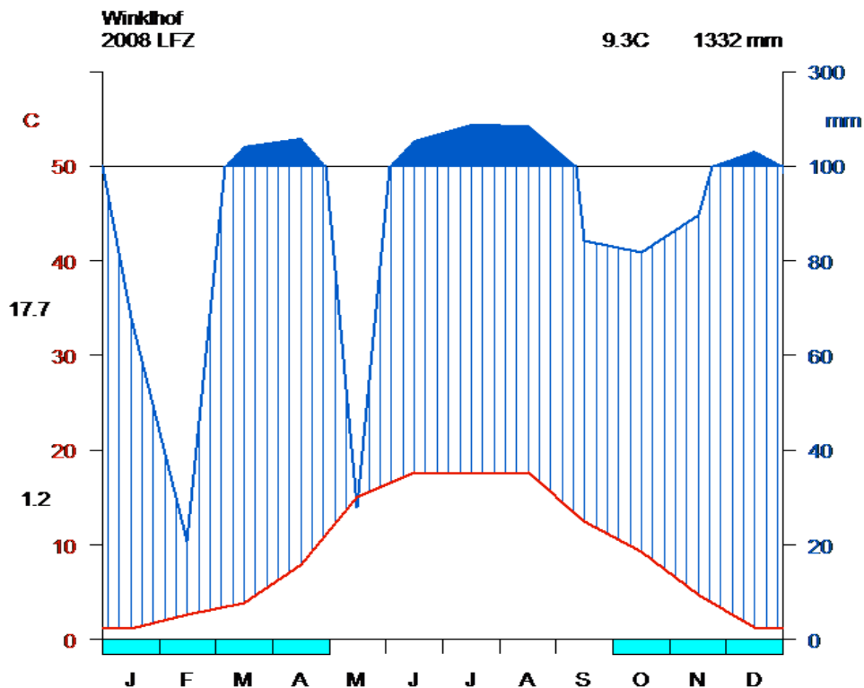
Abbildung 8: Klimadiagramm 2008
