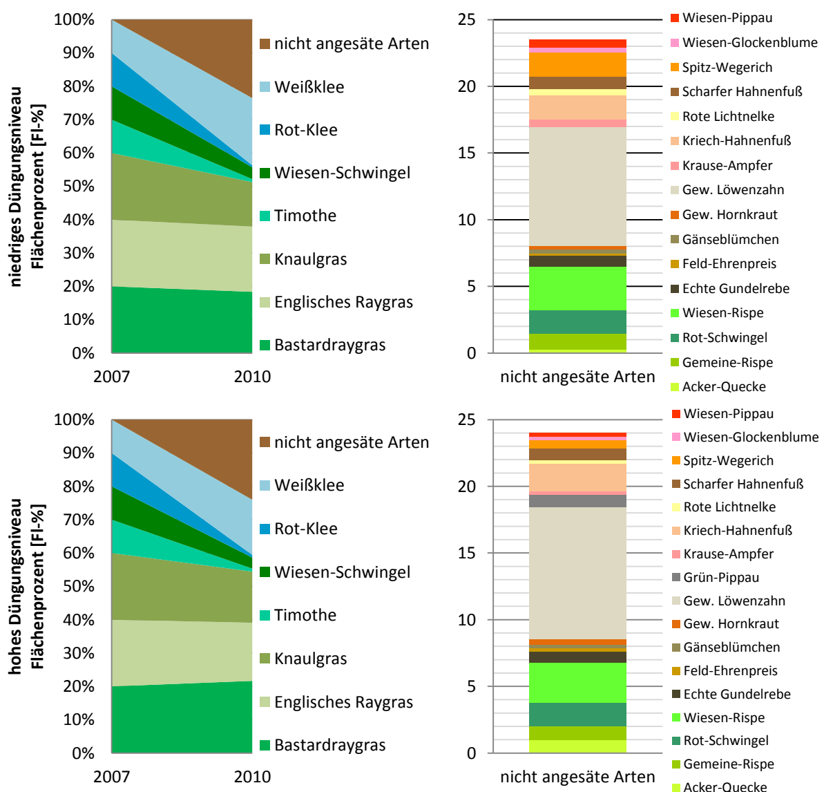
Abbildung 19: Entwicklung des Pflanzenbestandes auf den ohne Lysimetersystem ausgestatteten Parzellen des Lysimetervergleichsversuches Winklhof
