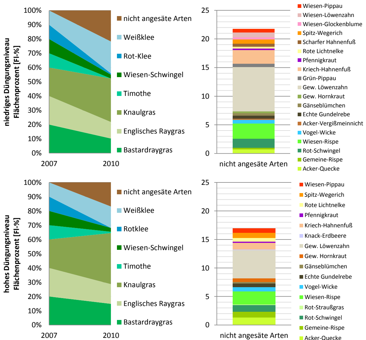
Abbildung 18: Entwicklung des Pflanzenbestandes auf den mit Schwerkraftlysimeter ausgestatteten Parzellen des Lysimetervergleichsversuches Winklhof
