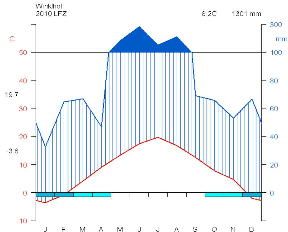
Abbildung 10: Klimadiagramm 2010
