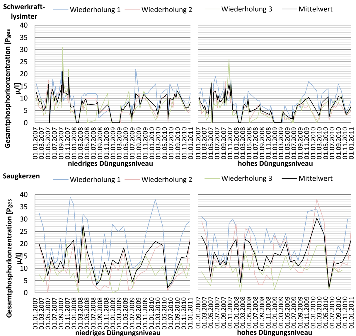
Abbildung 31: Verlauf der Gesamtposphorkonzentration im Sickerwasser über den gesamten Versuchszeitraum
